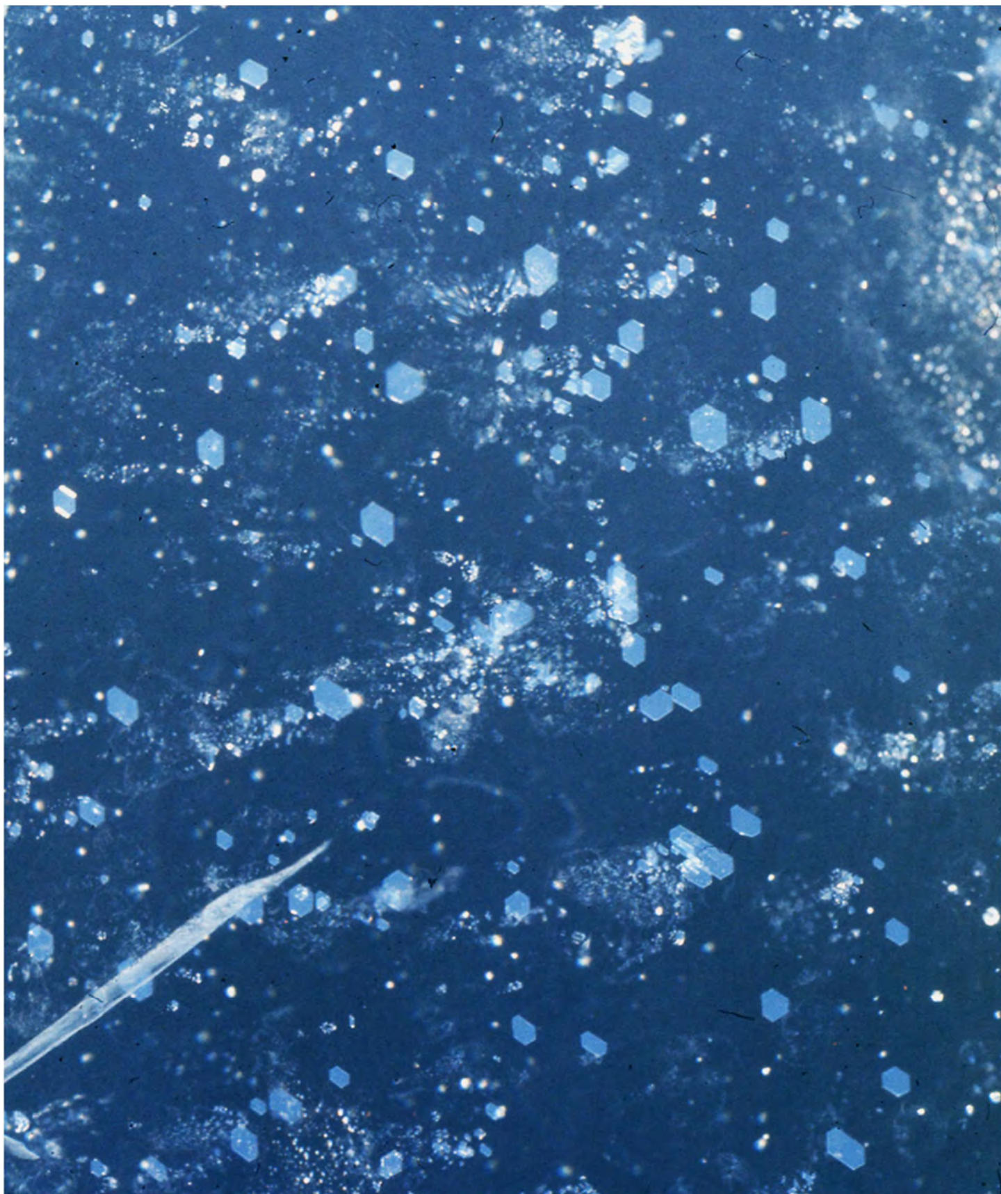
写真 154. 氷の中に散在する小さな「空像」(春採湖 1 月)。日射吸収のために氷内部に融解水が発生する。その融解水が再凍結するとき、氷と水の体積差から生じた真空の泡(水蒸気はある)が氷結晶中に残ったものが空像である 26) 。形は六角形である。
