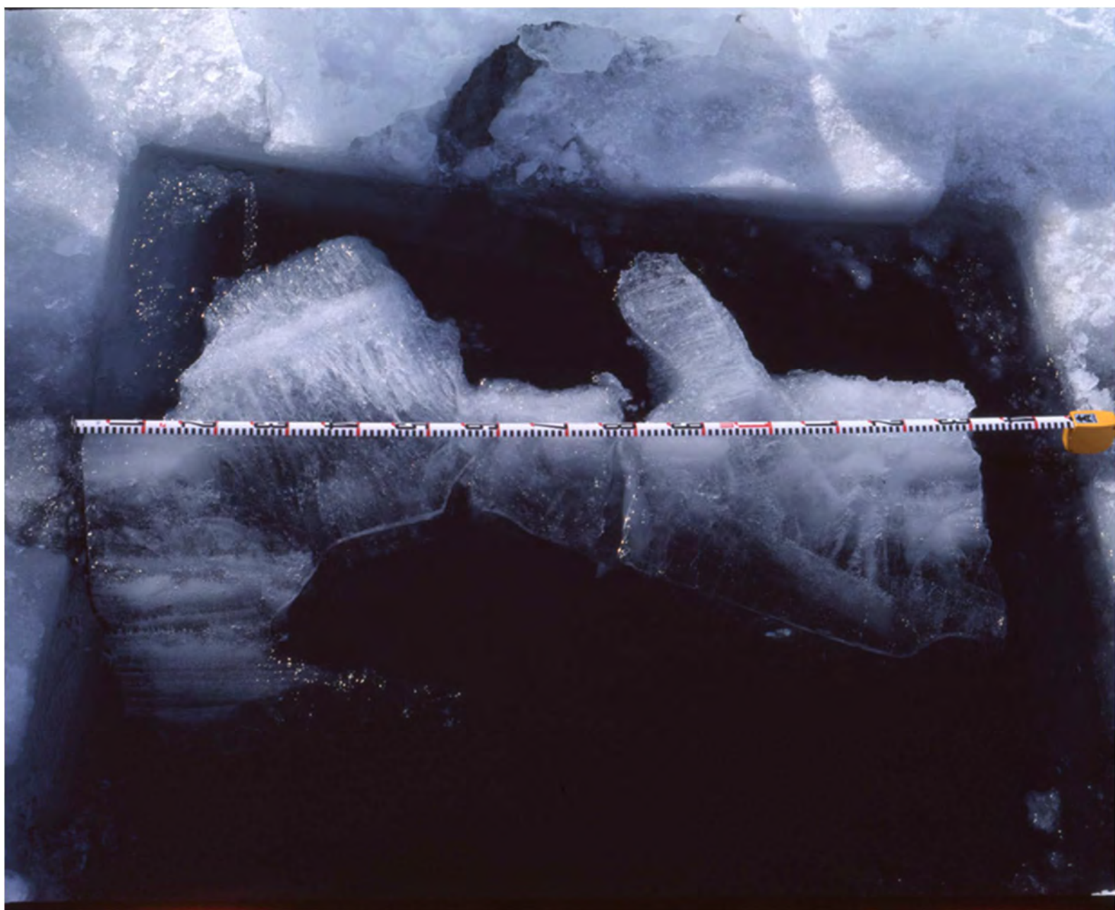
写真 131. 前の写真で切り出した御神渡りの断面 23) (屈斜路湖, 3 月)
