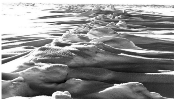
写真 175. Pressure Ice Ridge (北極海 T3 氷島 30) 付近)。風や海流などの外力によって隆起する (1973 年 5 月 9 日、河村章人氏撮影)。
