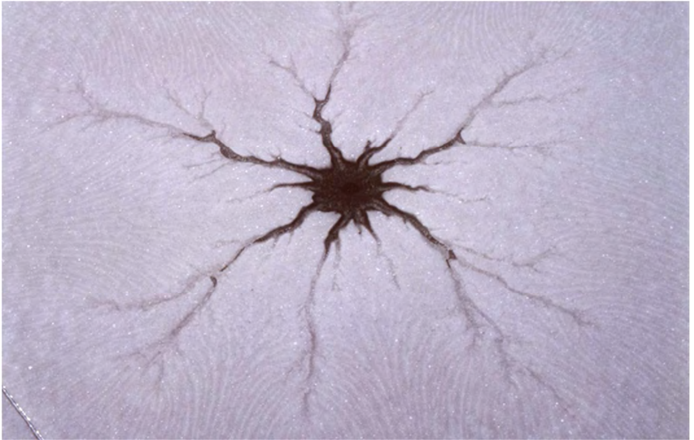
写真 80. 流線を示す氷紋(塘路湖、2 月)
