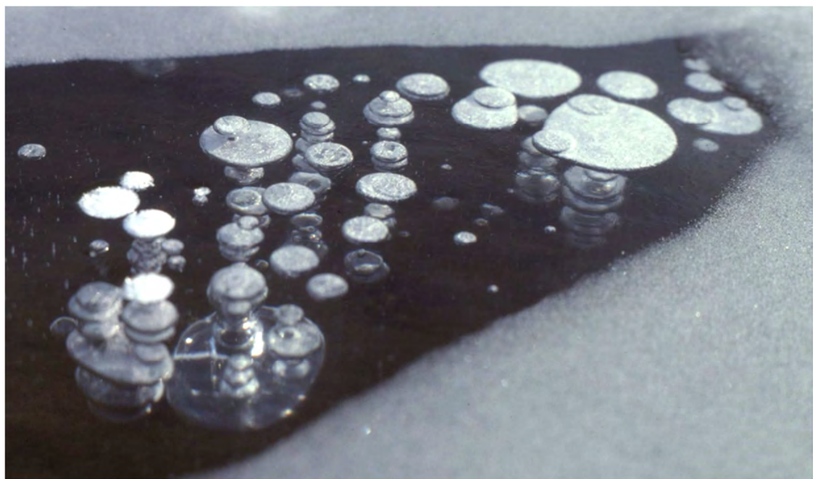
写真 90. いったん融解した氷が再凍結したときの気泡氷(塘路湖、2 月)
