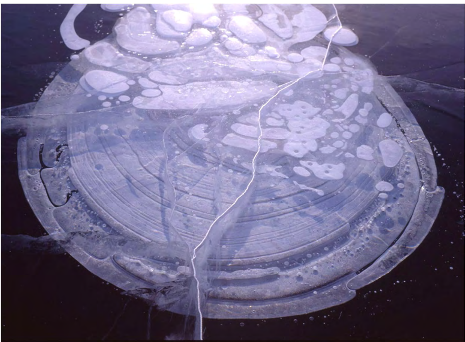
写真 92. 大きな泡の繊細な構造。巨大 UFO のようにも見える(シラルトロ湖、1 月)。
