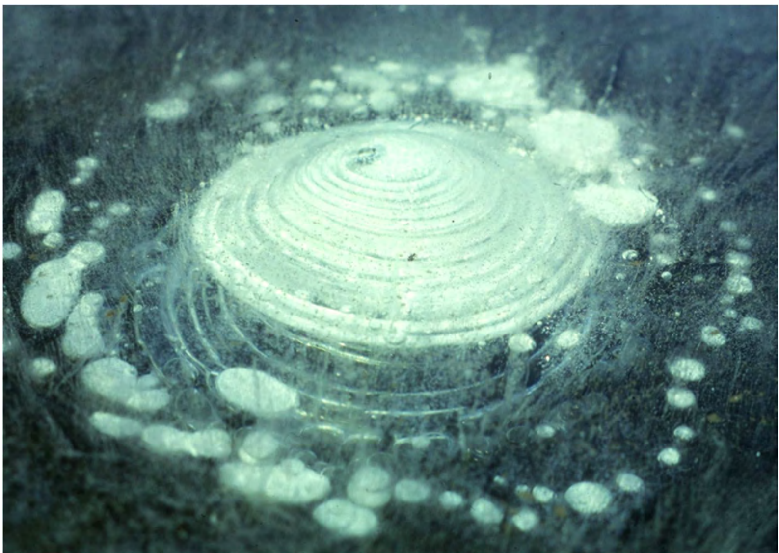
写真 95. 爆発した渦巻銀河？メタンガスが逆スリバチ状に蓄積した。穴をあけて点火すると炎が上がるがメタンガス濃度は 40%～70%と爆発濃度より濃いので危険は少ない（春採湖、1 月）。
