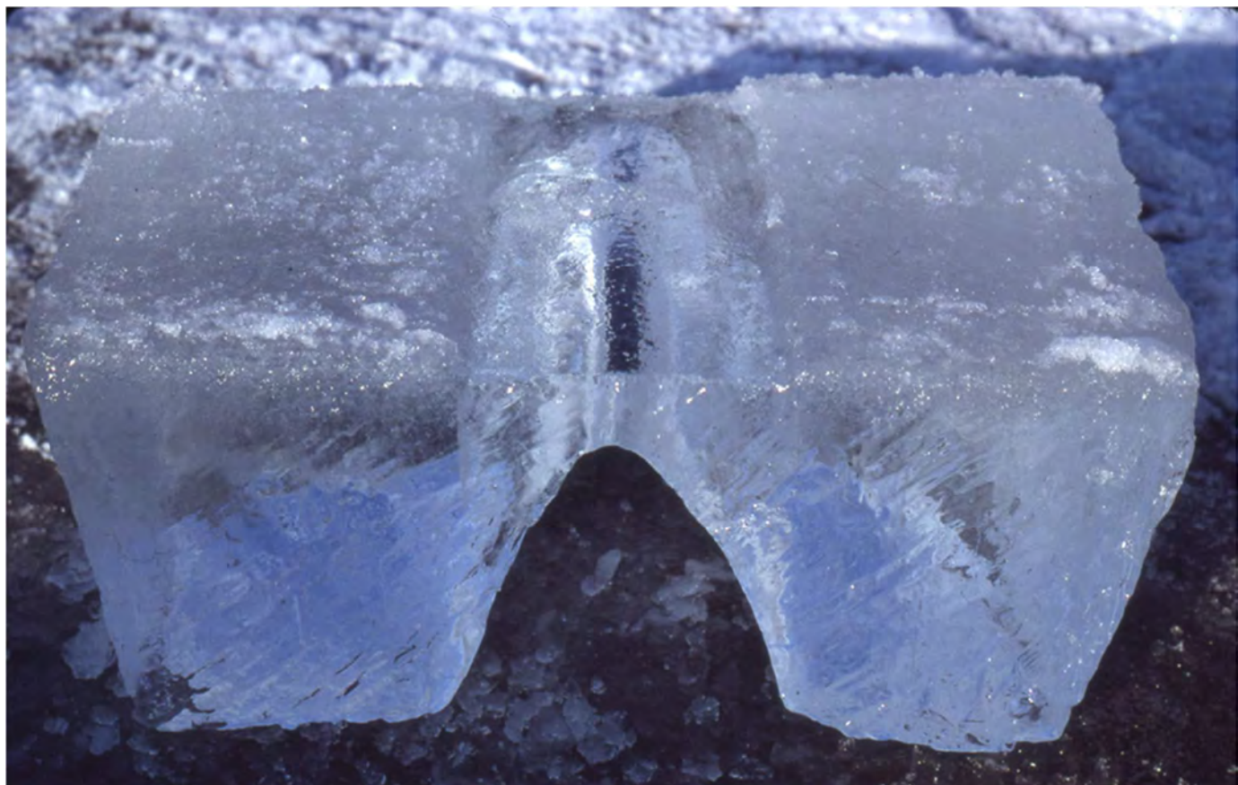
写真 132. 亀裂の断面。アーチ状に新しく氷が張り始めている。このような幅の広い亀裂で破壊が起り、御神渡りができ始める(屈斜路湖、2月)。
