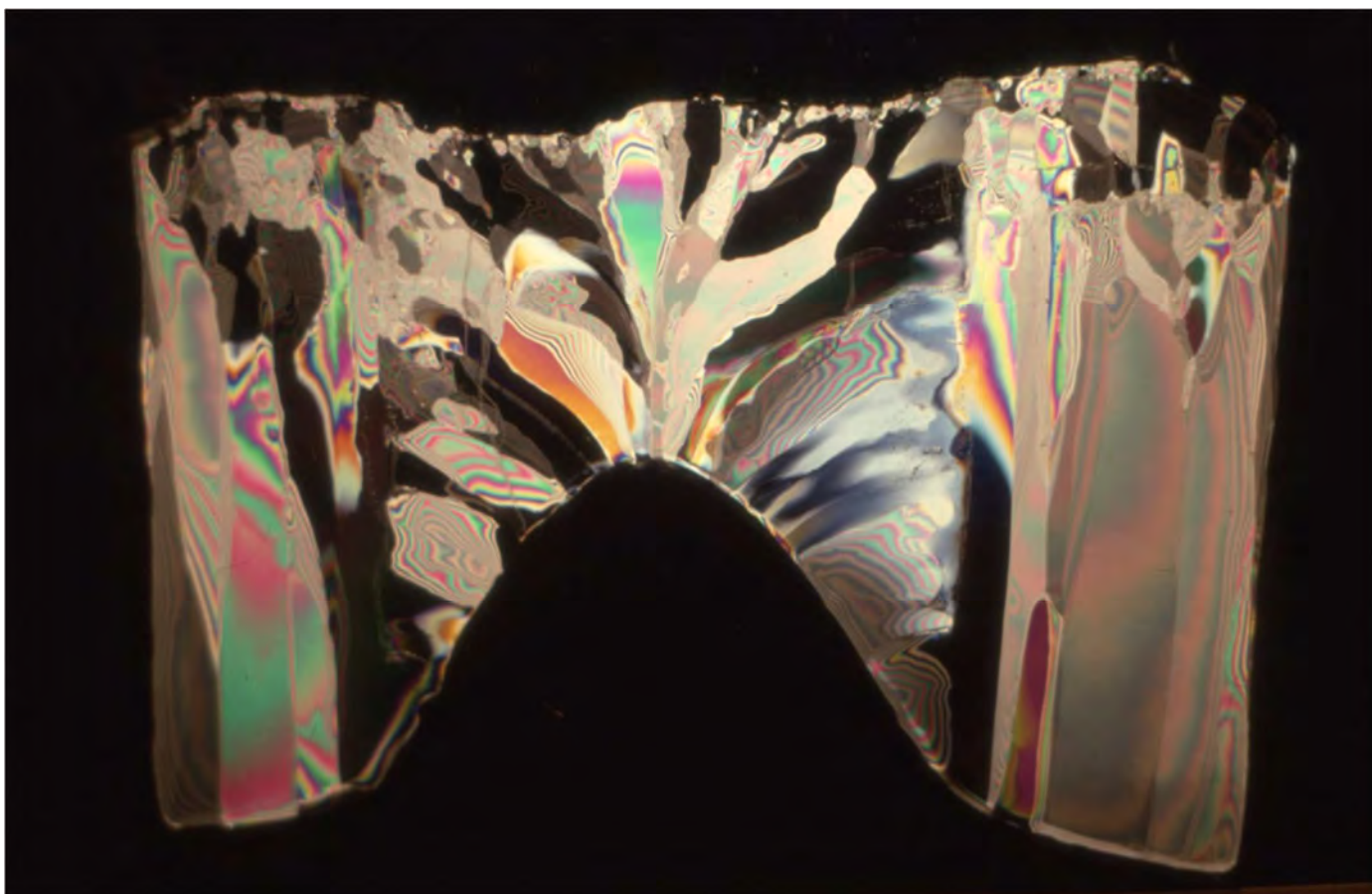
写真 133. 亀裂断面の偏光 24) 写真(屈斜路湖、2月)
