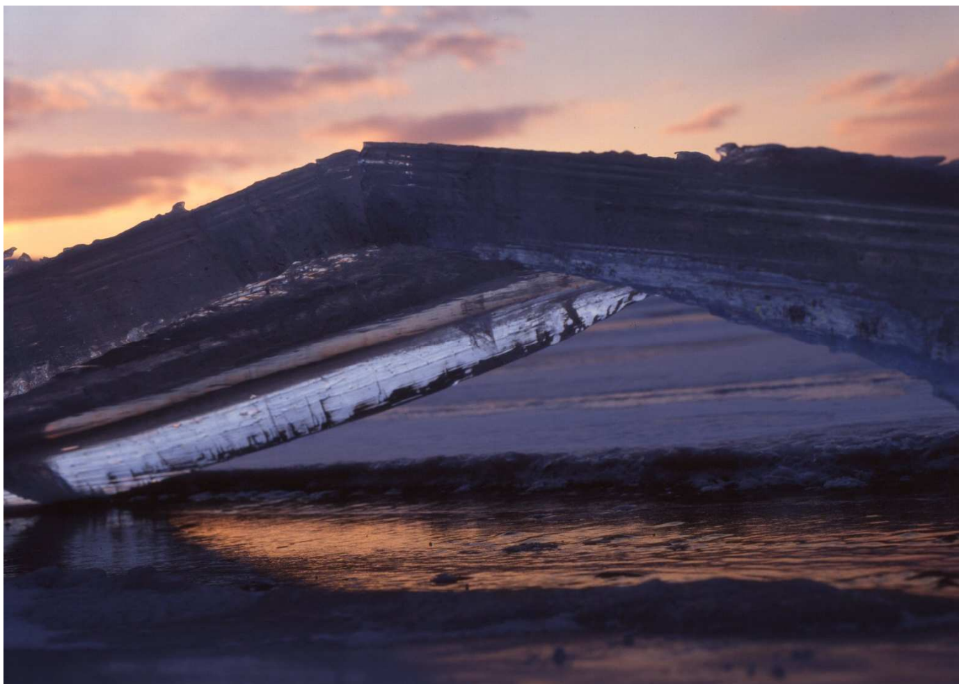
写真 140. 夕日に映えるアイスブリッジ(屈斜路湖、3月)。
