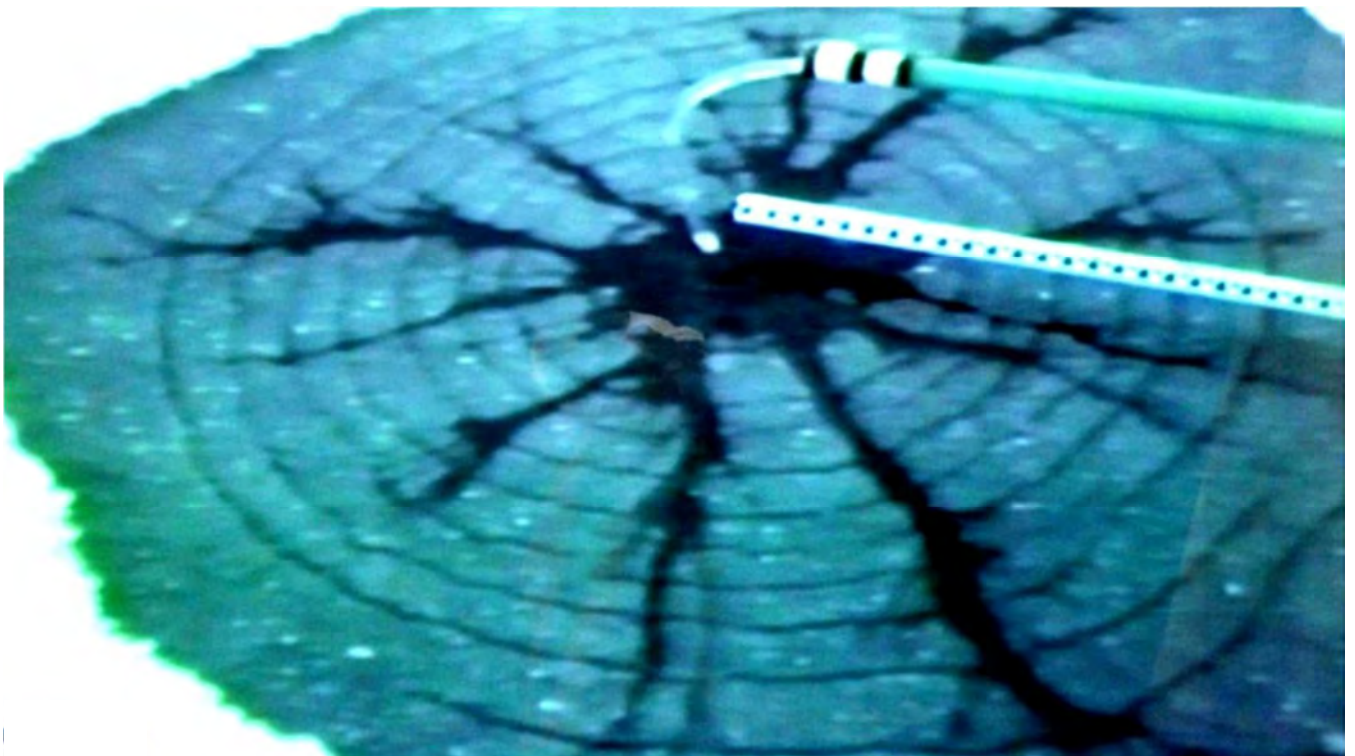
写真 149. 同心円氷紋作製世界第一号(春採湖、1984年1月1日)。世界で最初に人工作製に成功した同心円氷紋、これにより、形成機構の解明ができた。7章動画2参照。
