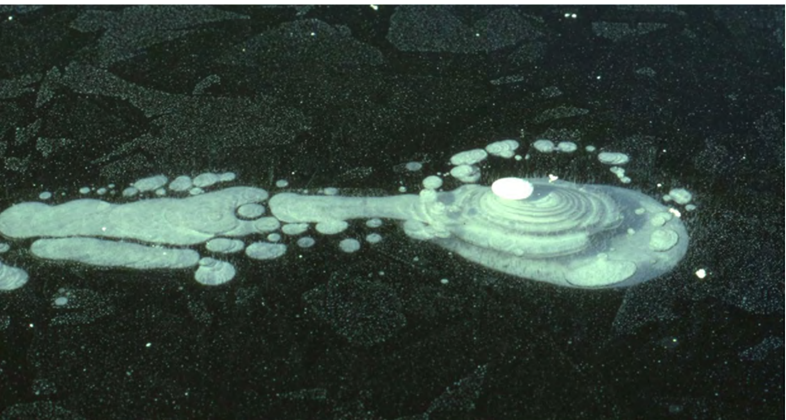
写真 89. 水平に広がったメタンガス(春採湖、12 月)
