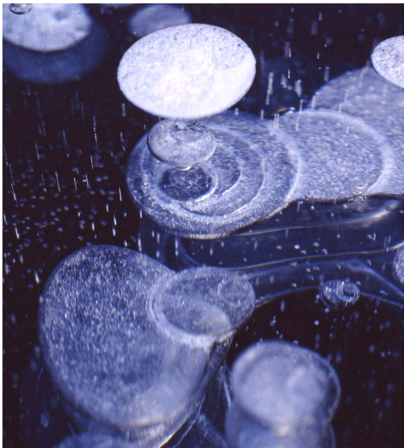
写真 87. 白い気泡氷。表面がよく冷える時、温度勾配による水蒸気移動のために、泡の天井側に霜が成長して白く見える。上の泡が白いのは、表面ほど温度勾配が大きかったことを示す。下部の泡は、まだ、霜の結晶が少ない(屈斜路湖、2 月)。
