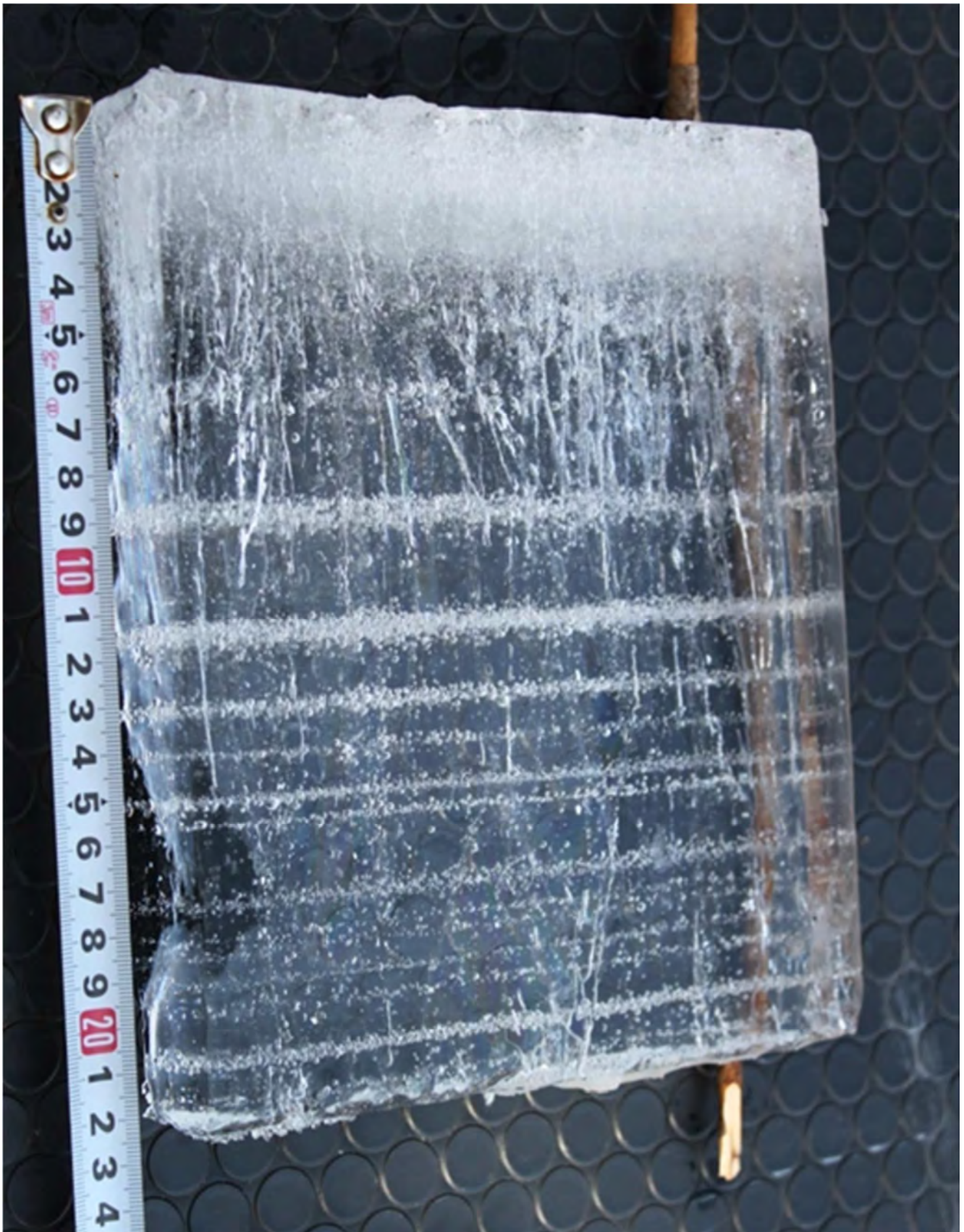
写真 153. 水深の浅い岸边に近い湖面の湖水断面。上部の白色部は積雪による氷、多数の水平縞は気泡層。この気泡は湖底藻類の光合成ガスによる酸素。湖底に日光が届かない水深の深い所での湖水では、このような気泡層はない(屈斜路湖、2019 年 4 月 1 日)。
