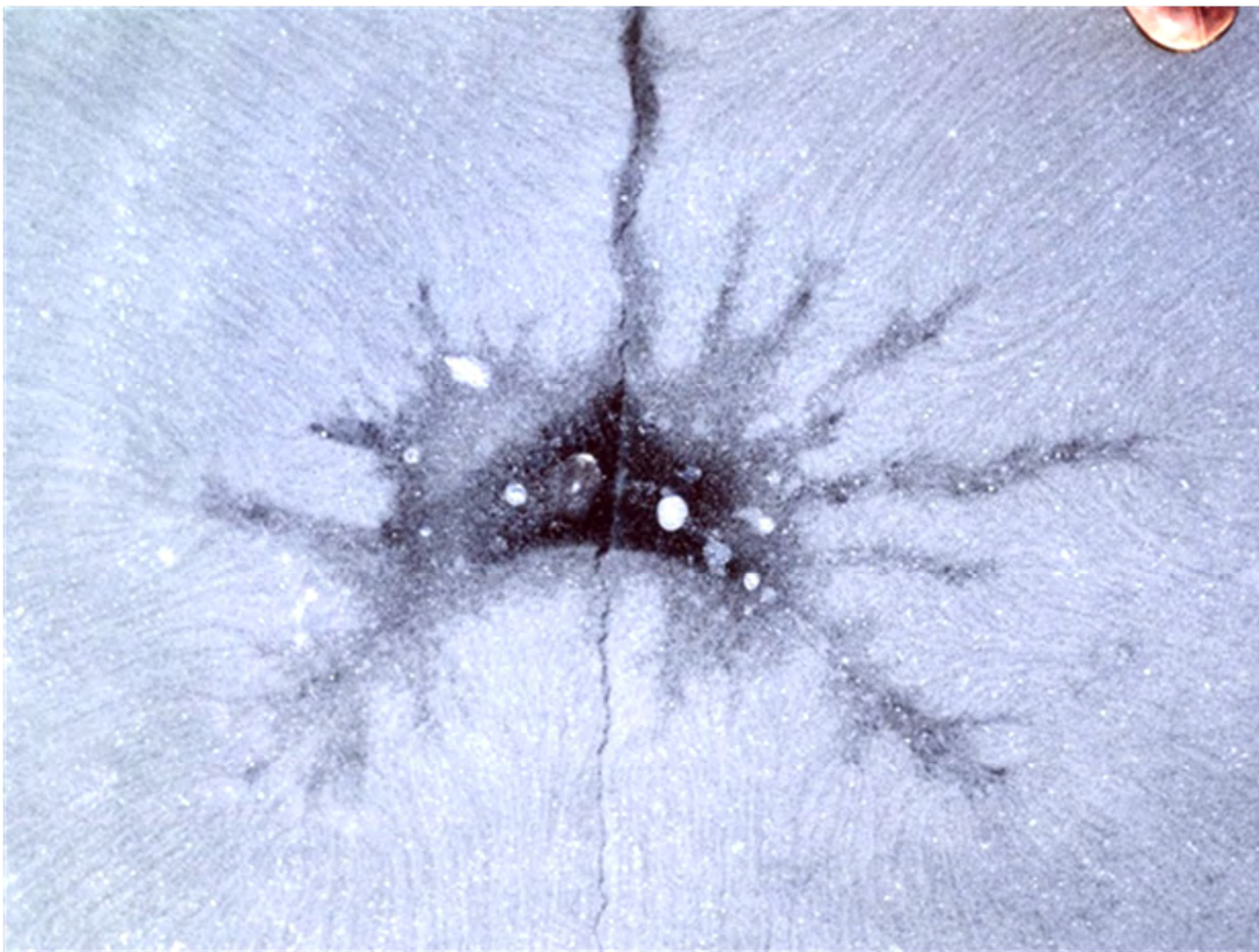
写真 79. 流線を示す氷紋(塘路湖、2 月)。放射状氷紋の周囲の雪面に 水の動きを示す流線が見える。
